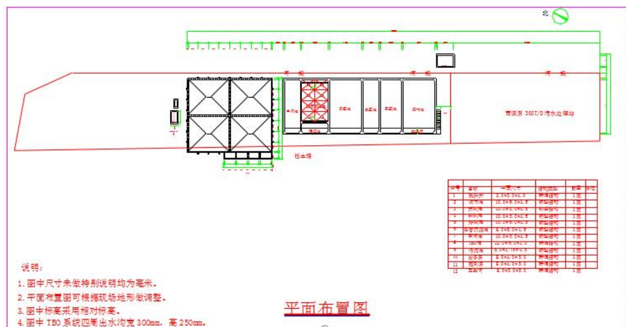
图3.3-2 现有污水处理厂平面布置图
