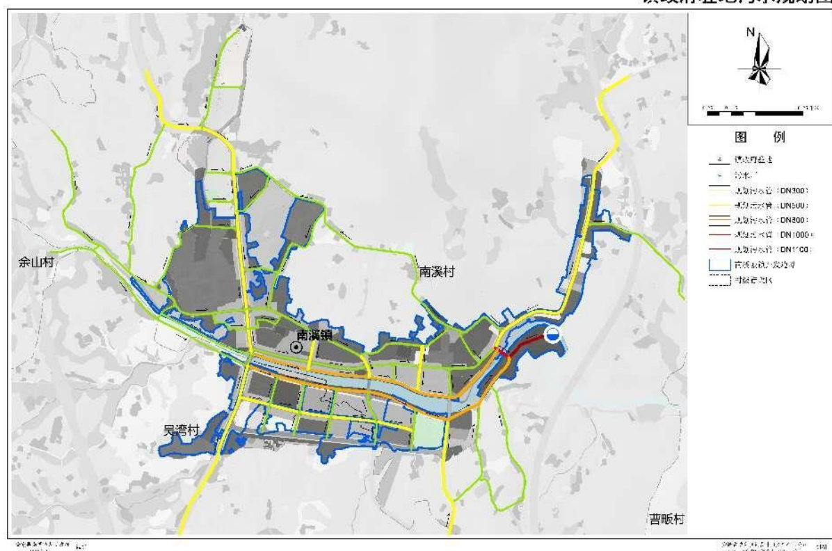
图 5.2-1 南溪镇污水管网系统图
