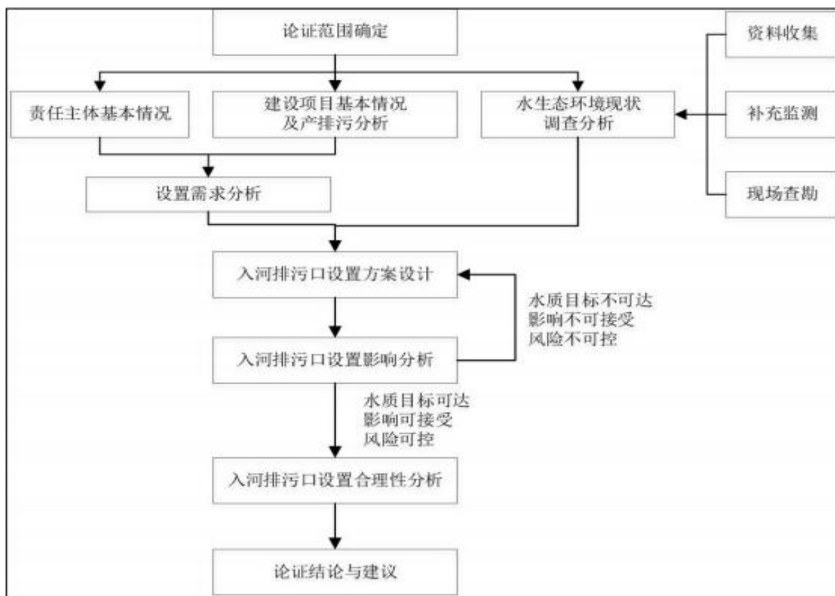
图1.4-1 论证工作程序框图
