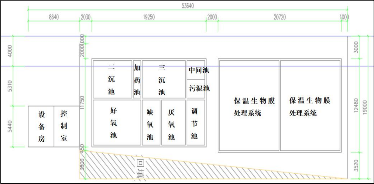
图3.3-3 南溪镇拟建1000t/d污水处理厂总平面图
