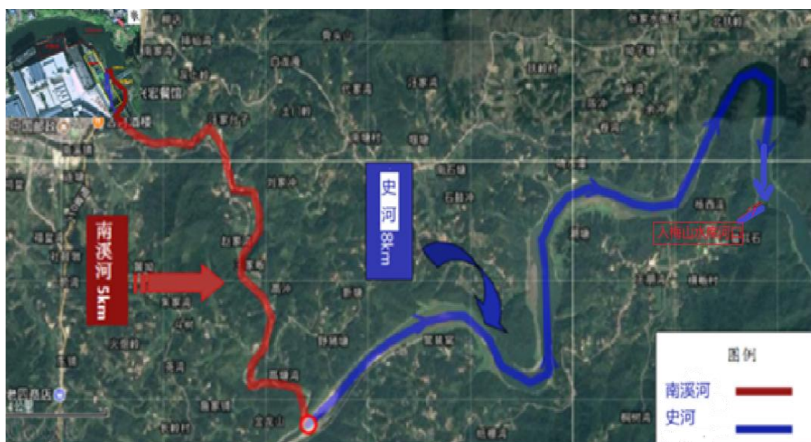
图 5.1-1 扩容项目排污口入河路线示意图
