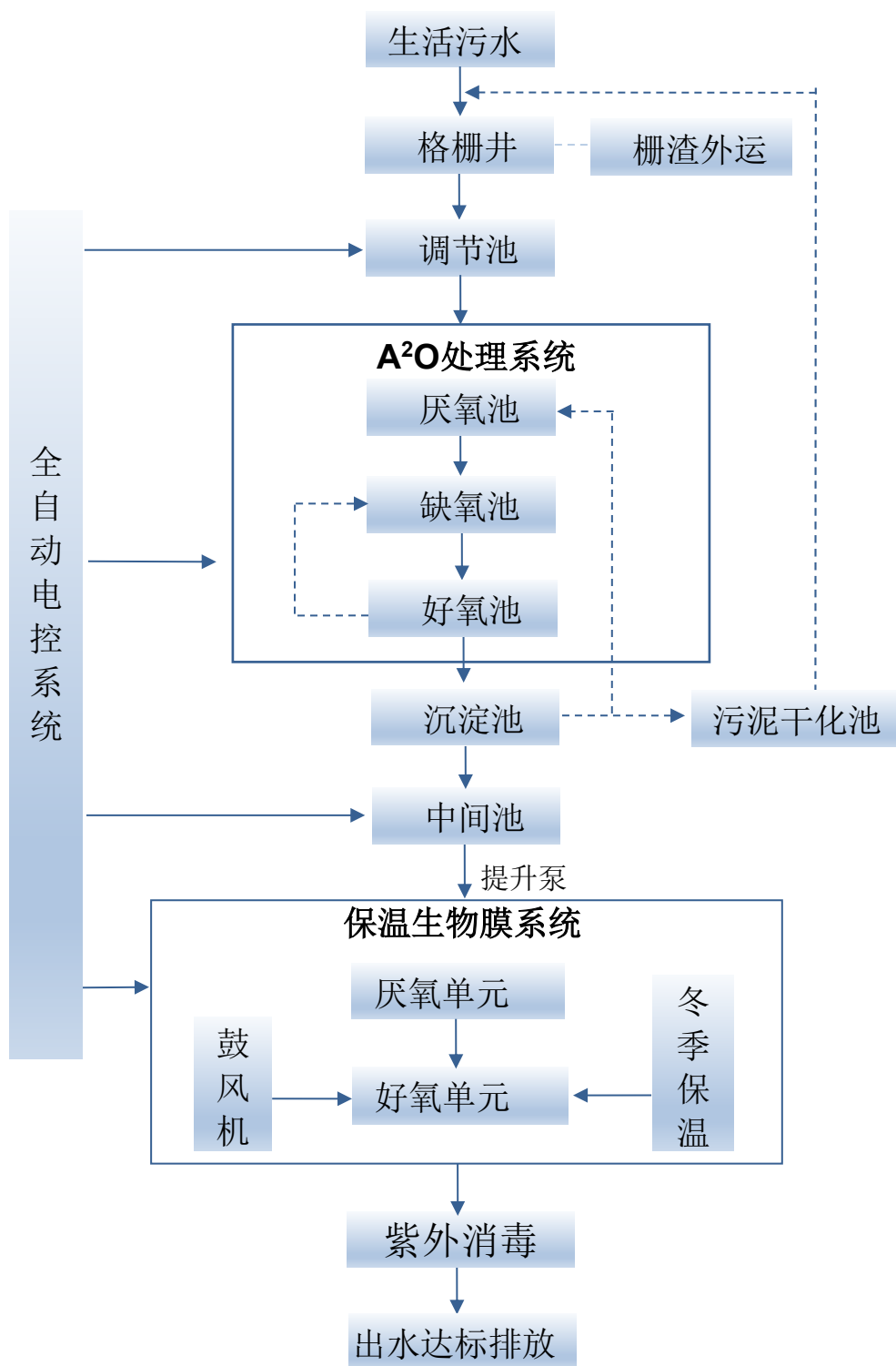
图3. 3-4 污水处理工艺流程
