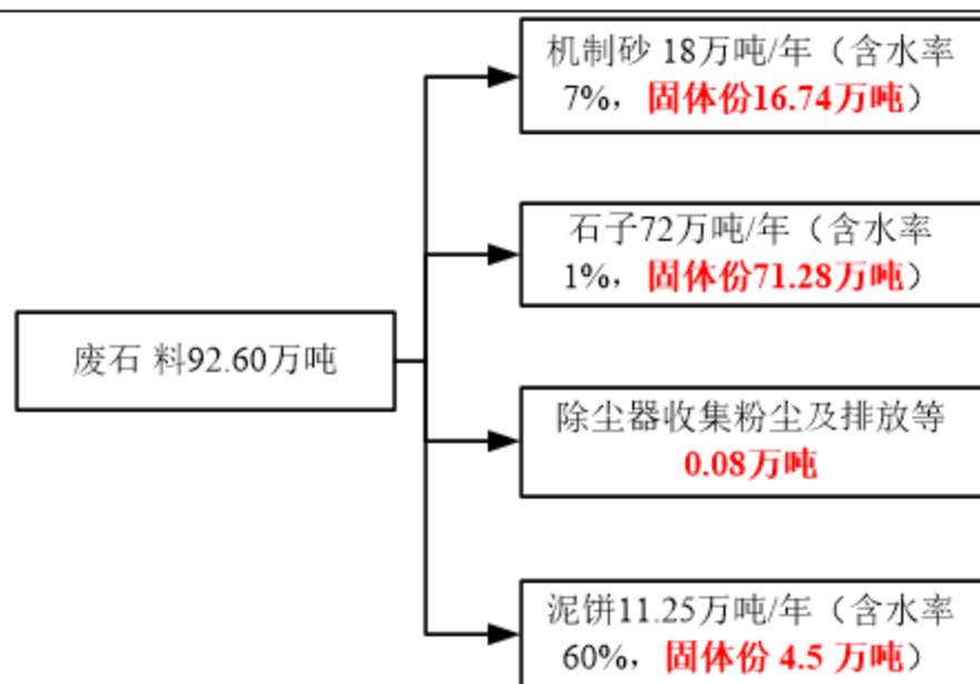
图 2-1 物料平衡图
