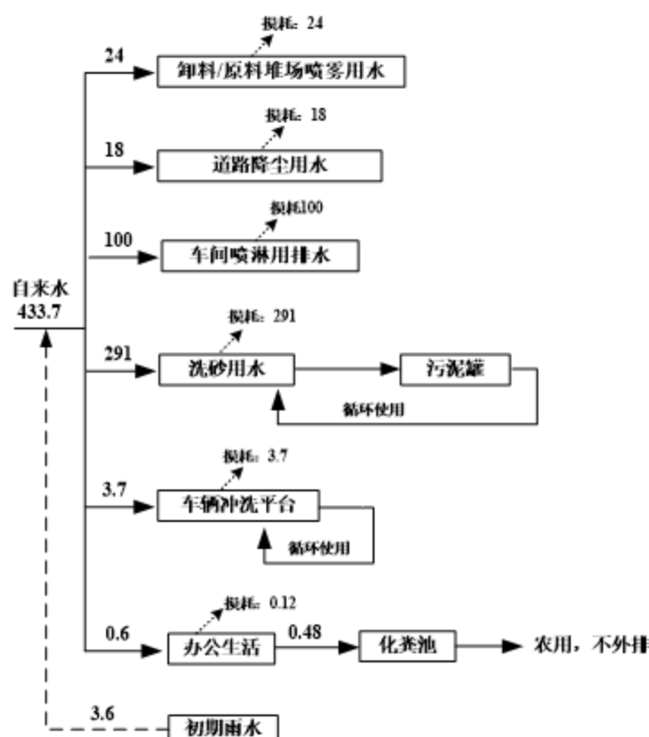
图 2-2 项目水平衡图 (t/d)
