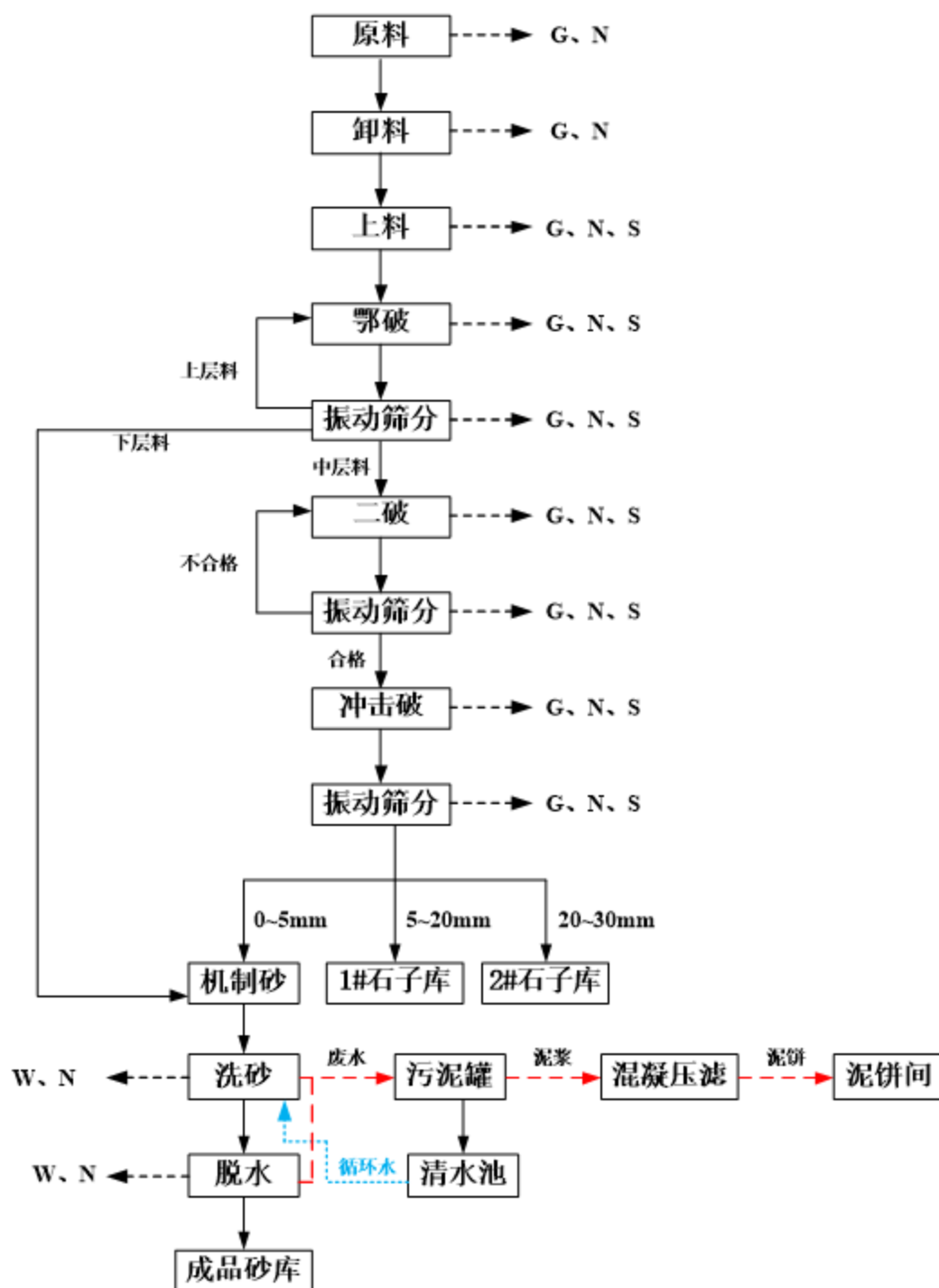
图 2-3 项目生产工艺流程及产污环节图
